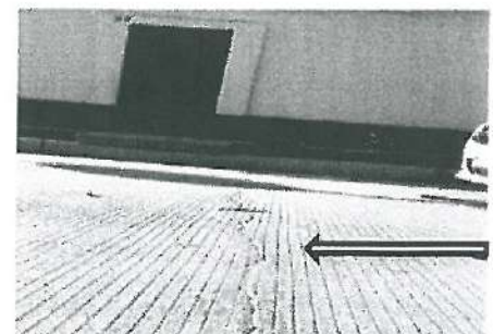
Se constato en la calle Gral. Ignacio Pesqueira se que presenta Mala calidad en la repararon de Gietas en la Losa de Concreto.
