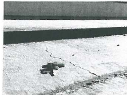
Grieta en Losa de Concreto de dimensión de 0.40 mts, en la calle Revolución entre calle 20 y calle 21.
