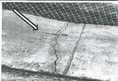
2 Grietas en Banqueta la cual tiene 1 metro lineal. C/u en la calle Ramon Teran (Frente de Iglesia)
