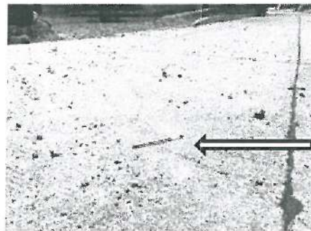
Grieta en Losa de Concreto de dimensión de 2.00 mts, en la esquina de las calles Brea y Sin Nombre.
