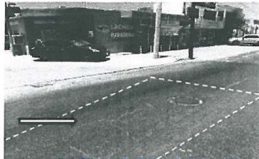
Grietas en Microcarpeta de 3.0 cm de espesor. Ubicadas enfrente de Panaderia La Chida
