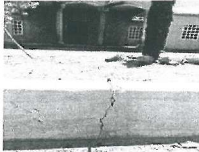
Grieta en Guarnición no.2
