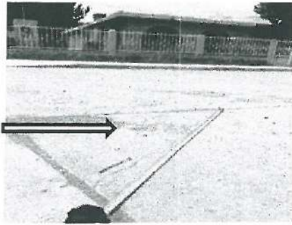
Grieta en Losa de Concreto de dimensión de 1.30 mts, en la esquina de las calles 21 de Marzo y Periferico.
