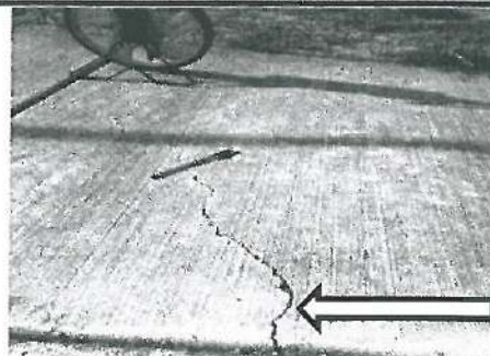
Grieta en Banqueta la cual tiene 1 metro lineal, Ubicada en esquina de calle Jose M. Leyva y Bacoachi.
