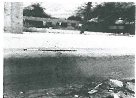
Grieta en Guarnición, en la esquina de las calles Sin Nombre y Callejon Sin Nombre.
