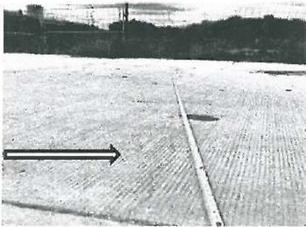
3 Grieta en Losa de Concreto de dimensión de 3.00 mts c/u, en la calle 21 de marzo entre Sexta y Kaly Mungaray.
