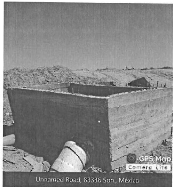
Construcción de caja de llegada de emisor a base de concreto y acero.
