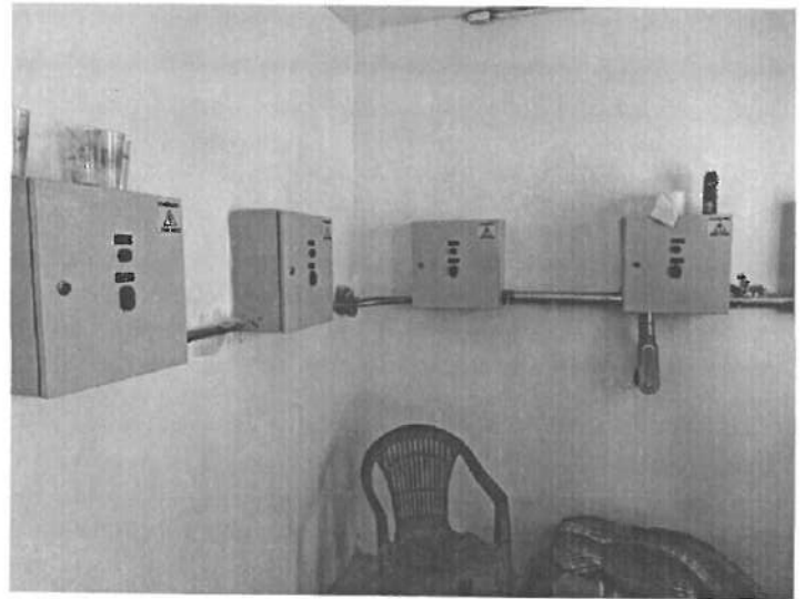
Colocacion de alimentador de centro de carga a transfer planta de emergencia
