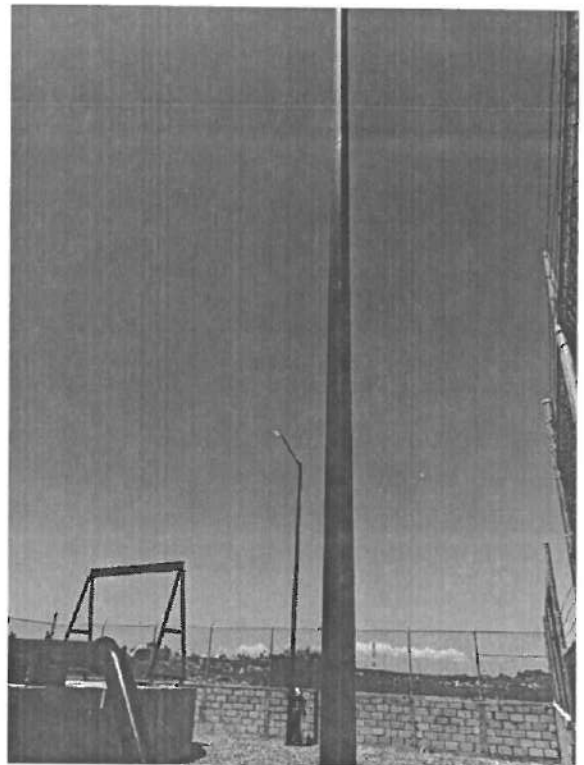
Colocacion de base prefabricada de concreto 70X60X40, colocacion de poste cónico circular de 8 mts, instalación de luminaria led de 80 watts
