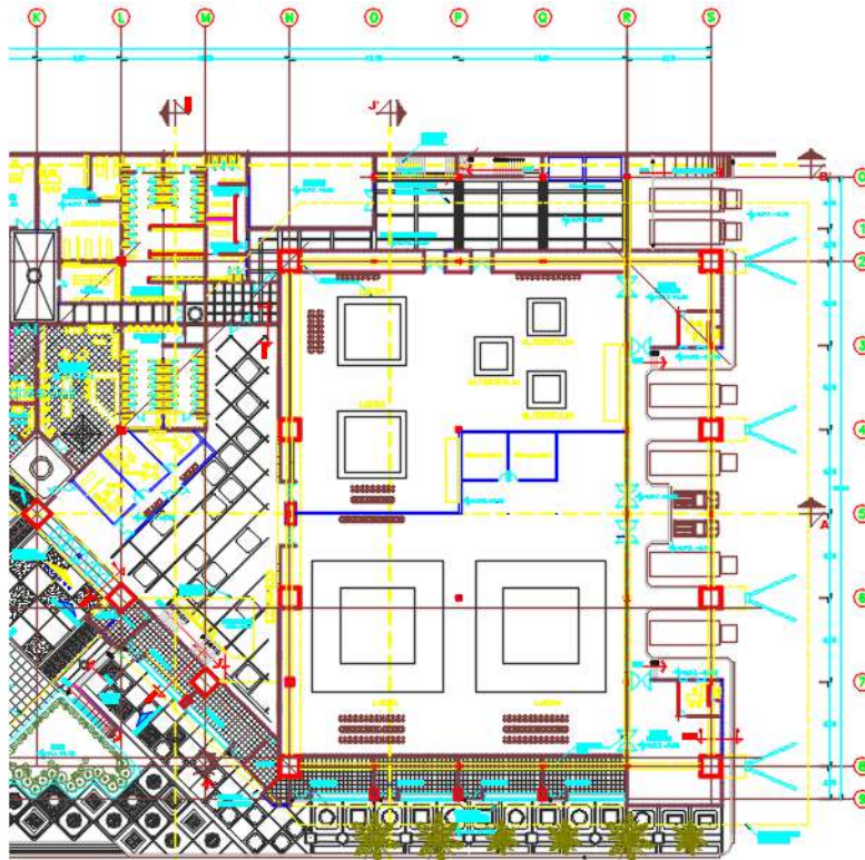
Anteproyecto Planta Baja, Distribución de Áreas
