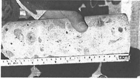
Etapa de presentación de Extracción, con datos de ubicación de la Carpeta de Concreto Hidráulico de los cadeneramientos 2+850
