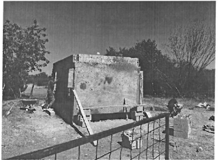
COLOCACIÓN DE MORTERO EN MUROS DE DORMITORIO
