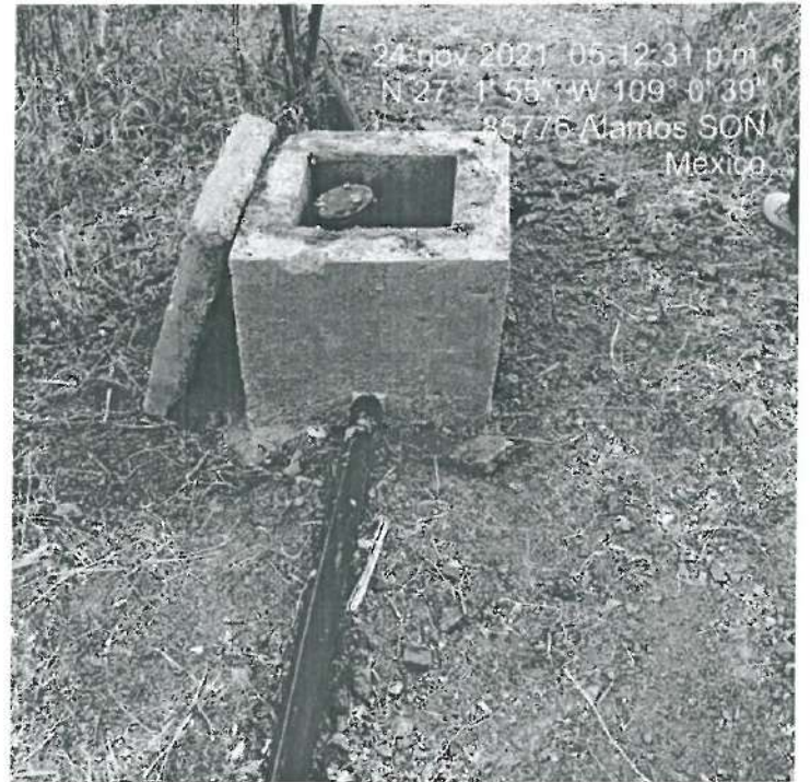
VISTA DE REGISTRO DE VÁLVULA DE ADMISIÓN Y
