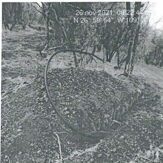
VISTA DE ZANJA Y COLOCACIÓN DE TUBERÍA DE PVC DE 2"
