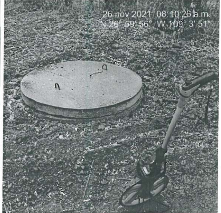
VISTA DE REGISTRO PARA VALVULAS DE ALIVIO
