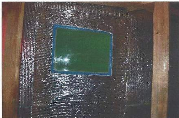
Suministro e instalación de ventanilla de cristal con marco de fibra de vidrio, instalación de aislamiento reflectix en tanques de reproductores.
