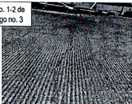
Hallazgo no. 3 Estacionamiento en Lado Oriente, Grieta que cubre 9 M2 de Superficie de Losa de Concreto.
