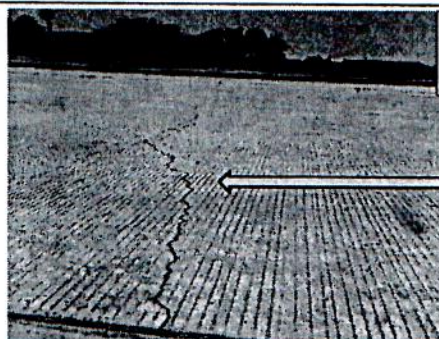
Hallazgo no. 4 Estacionamiento, en la Entrada al Acceso de Ambulancias Grieta que cubre 9 M2 de Superficie de Losa de Concreto.
