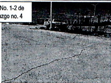
Hallazgo no. 4 Estacionamiento, en la Entrada al Acceso de Ambulancias Grieta que cubre 9 M2 de Superficie de Losa de Concreto.
