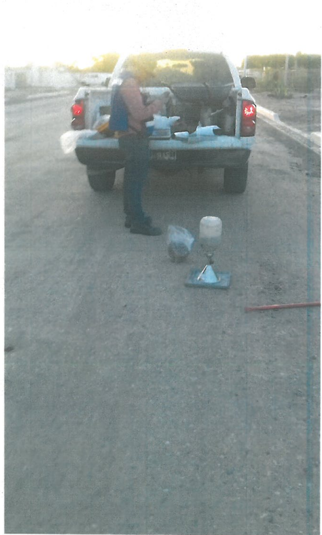
Muestreo de capa de sub-base para determinar su calidad y la realización de pruebas de compactación con el método de cono y arena.
