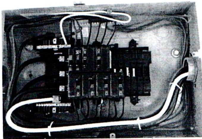
Centro de carga y termo magnéticos
