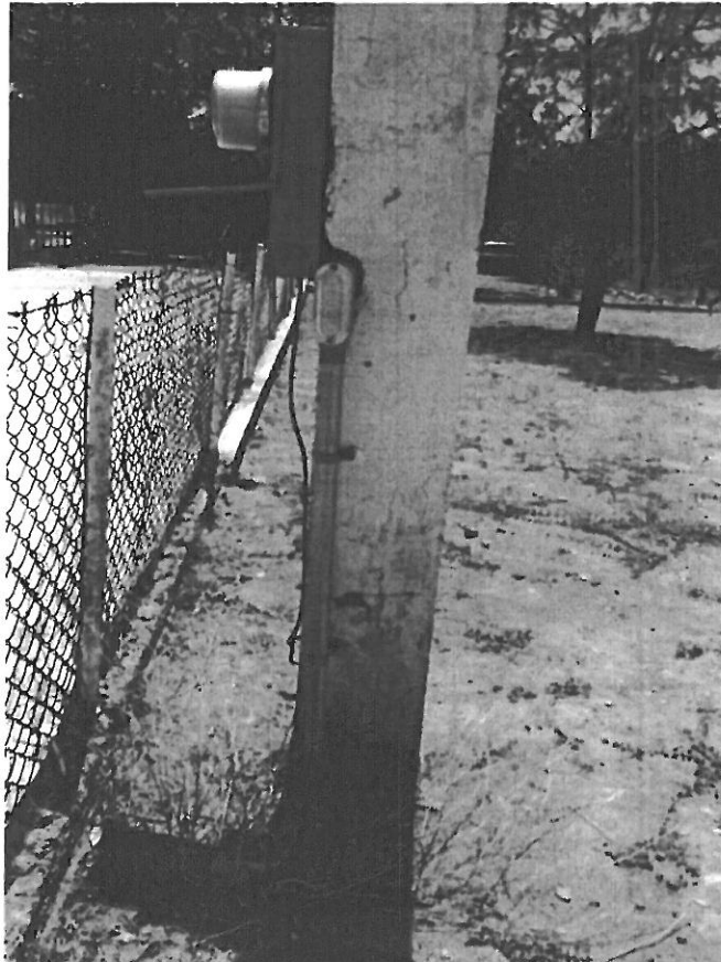
Interruptor principal y base de medición en gabinete Nema.
