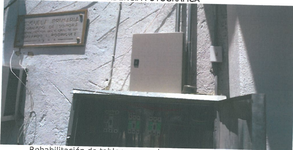
Rehabilitación de tablero general y centro de carga de 8 circuitos.
