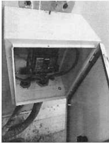
Fotografías que muestran el interruptor y el gabinete nema 3R, falla eliminada.
